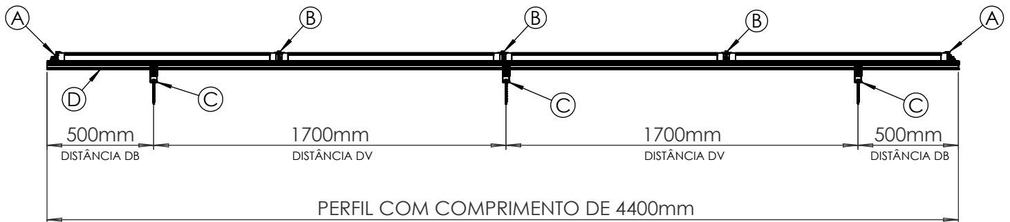
FIGURA 2 - VISTA LATERAL DA ESTRUTURA
