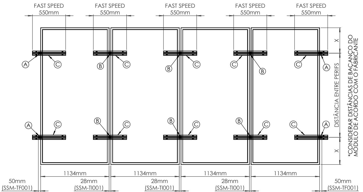
FIGURA 2 - VISTA SUPERIOR DA ESTRUTURA
