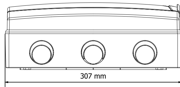
VISTA INFERIOR
